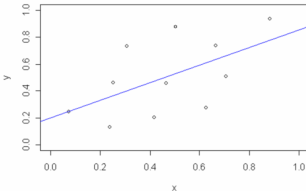
Figura 1. Diagrama de dispersión y recta ajustada
