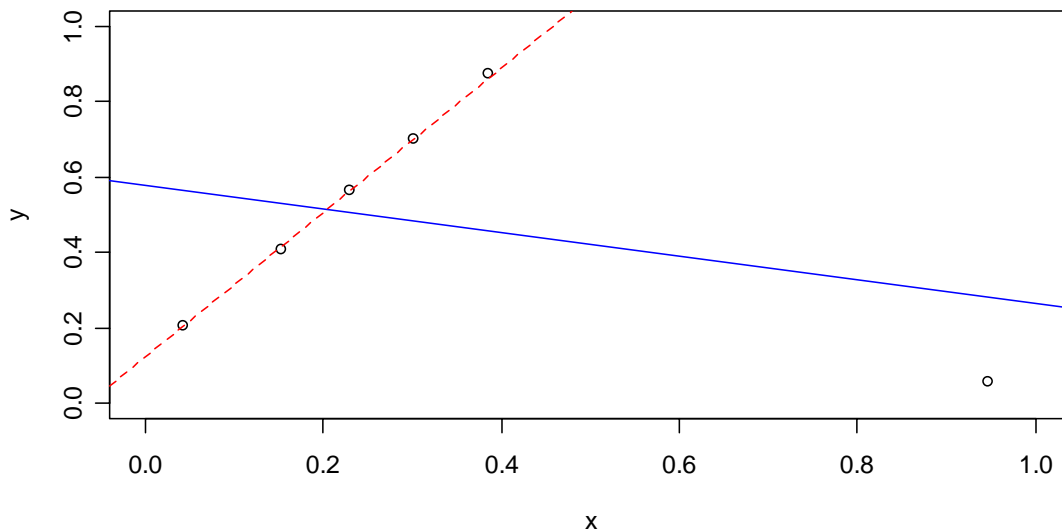
Figura 2. Recta de Cuadrados Mínimos y Recta Resistente
