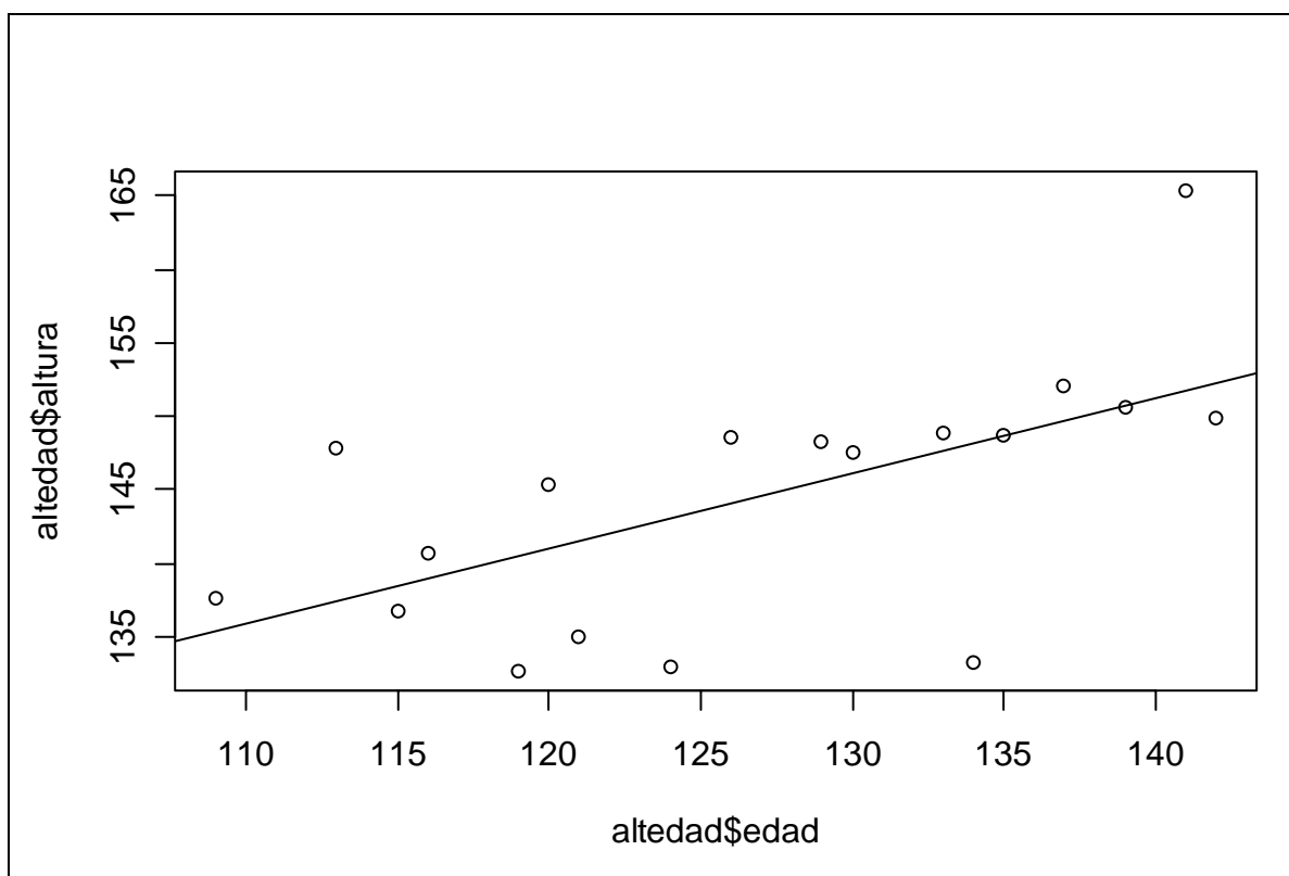
Figura 4. Recta de Cuadrados Mínimos
