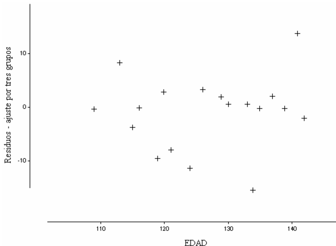
Figura 10. Residuos de altura vs. edad después de un ajuste iterado por tres grupos
