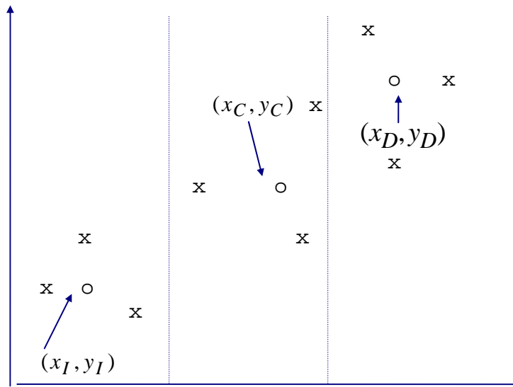
Figura 9: Los datos (x) y los puntos centrales (o) en un ejemplo hipotético.
