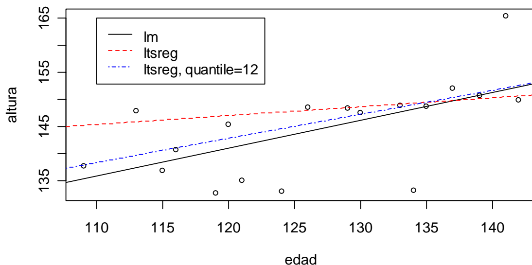
Figura 7. Comparación de tres ajustes
