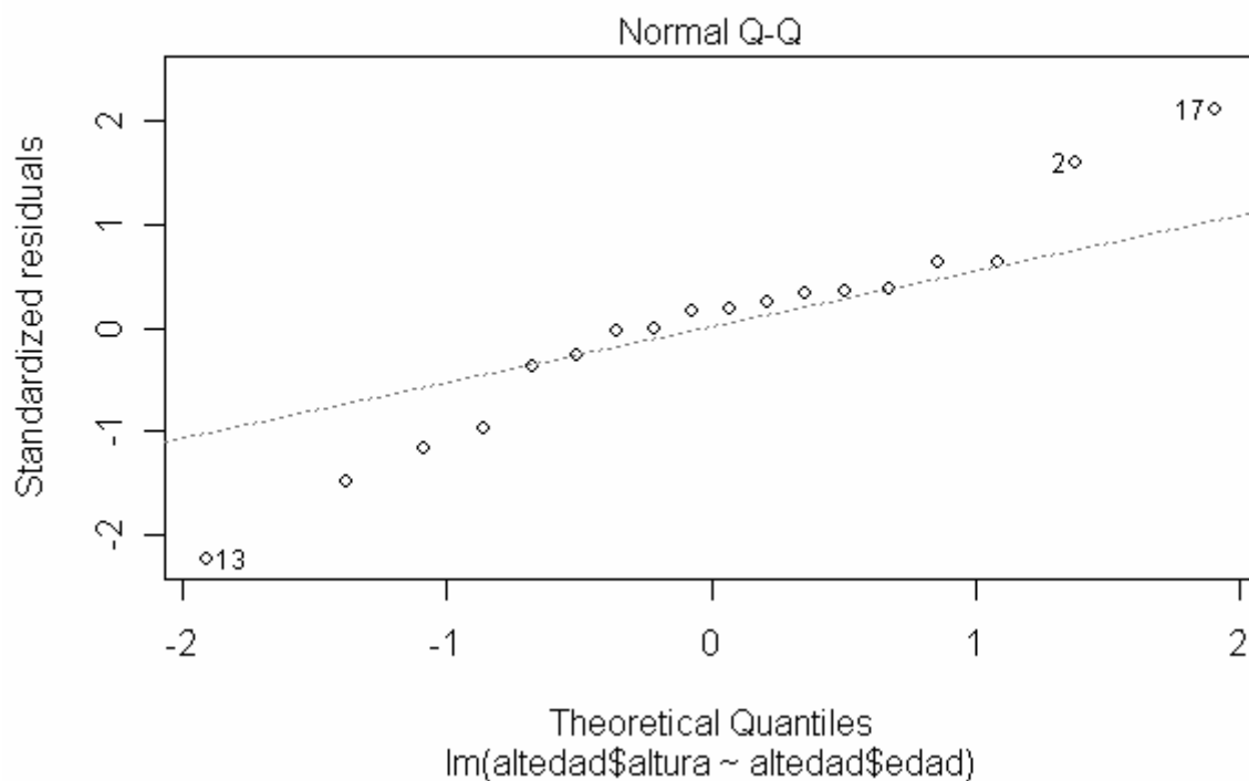
Figura 6. Gráfico cuantil-cuantil de los residuos, también se destacan los puntos 2, 13 y 17.
