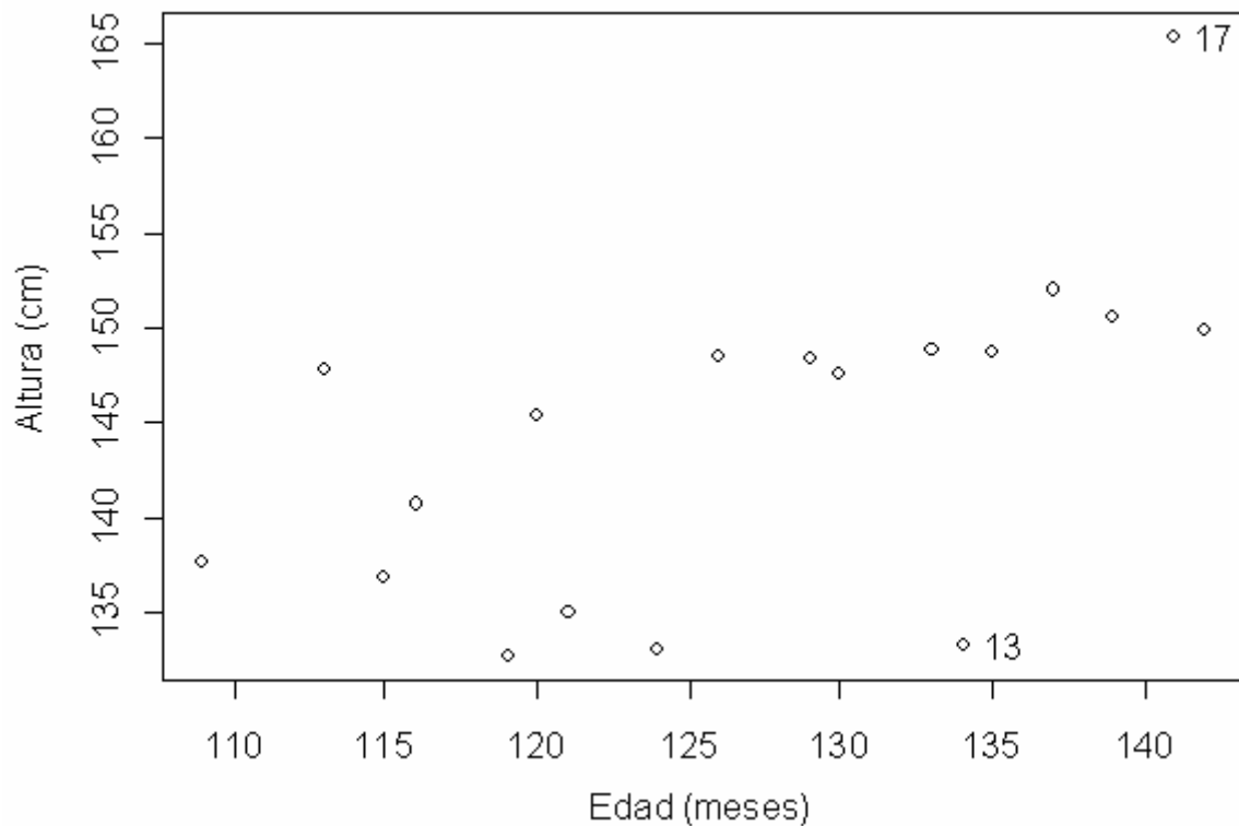
Figura 3. Diagrama de dispersión de altura vs. edad
