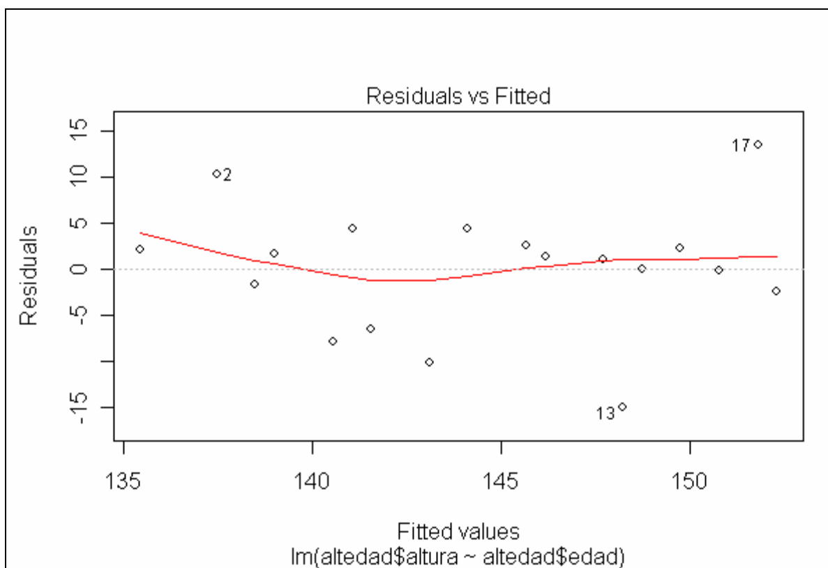
Figura 5. Residuos del ajuste de cuadrados mínimos
