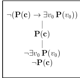
Figura 2.3: Árbol cerrado de \neg(\mathbf{P}(\mathbf{c}) \rightarrow \exists v_0 \mathbf{P}(v_0))
